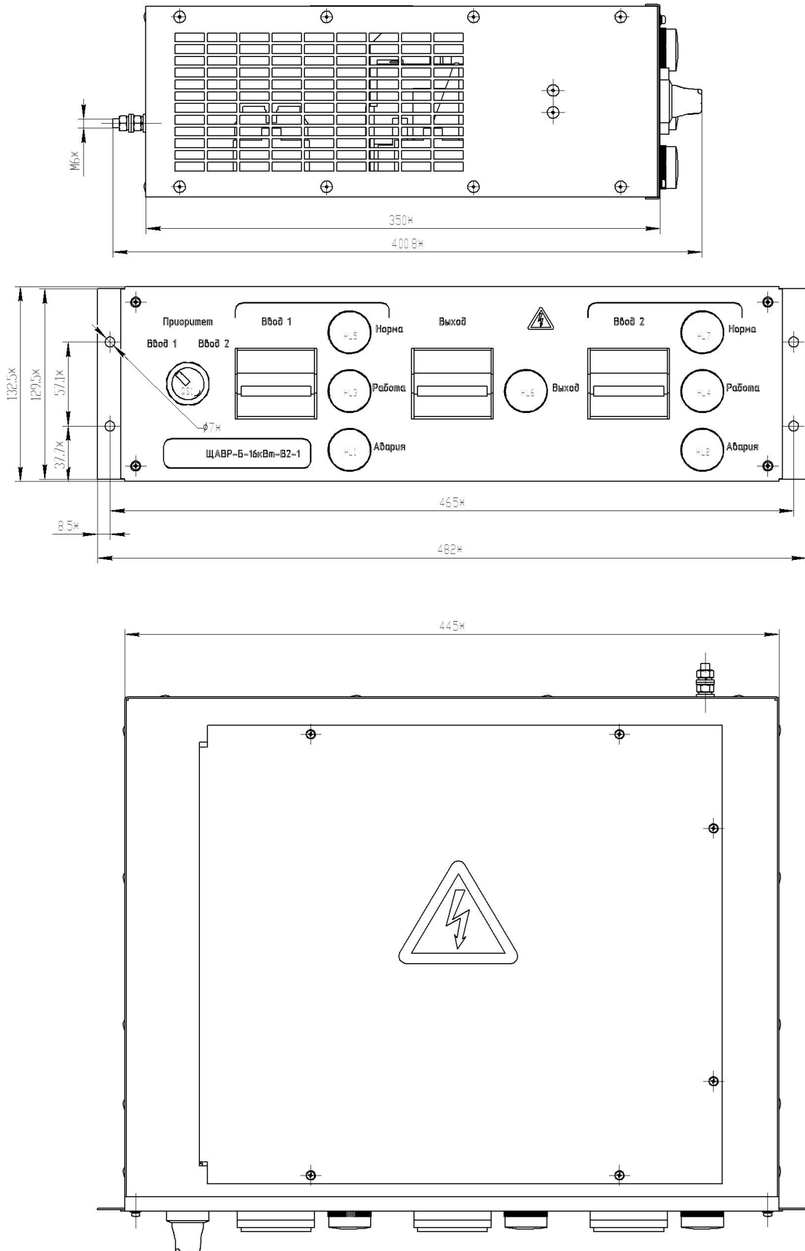
Рис.1. Габаритно-присоединительные размеры щита автоматического включения резерва ЩАВР-Б-16кВт-В2-1.
